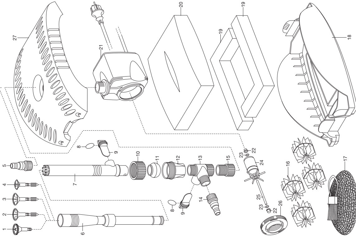
GARDENA Teichfilter mit Wasserpumpen-Set FFP 3000 Art.-Nr. 7887
