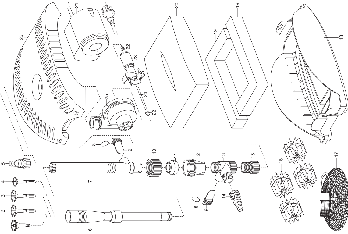
GARDENA Teichfilter mit Wasserpumpen-Set FFP 5000 Art.-Nr. 7888
