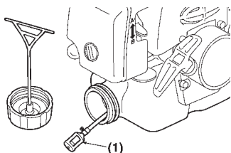
(1) Filtro del carburante
