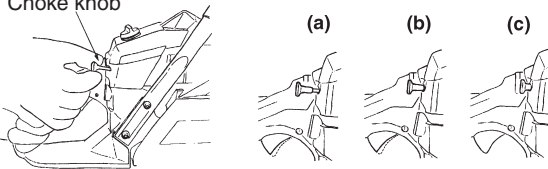
Choke knob
